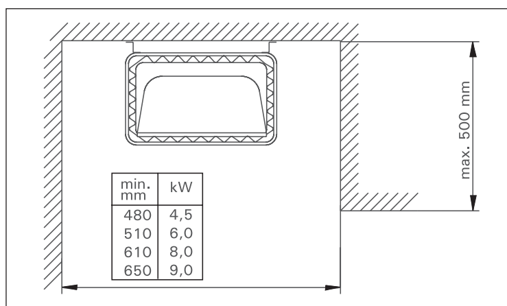
Figuur 2. De saunaoven in een nis installeren
