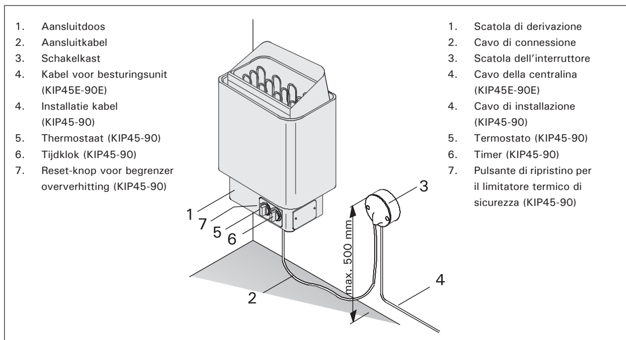
Figuur 1. Verbindingen en onderdelen van de saunaoven
